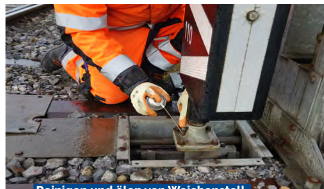
Reinigen und ölen von Weichenstellböcken und Signalen
