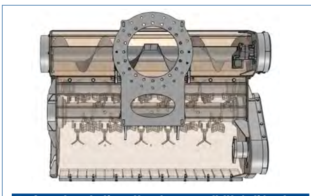
En fonction de l'application, possibilité d'équiper l'arbre de rotor avec différents couteaux
