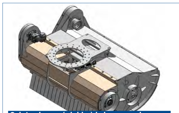
Galet palpeur réglable à la longueur de coupe souhaitée
