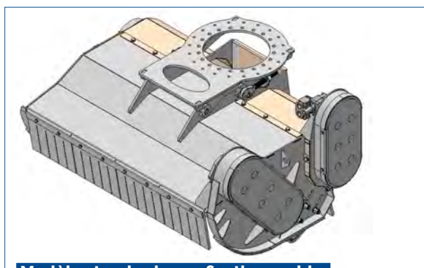
Modèle standard avec fixation rapide, avec châssis abaissé et robuste
